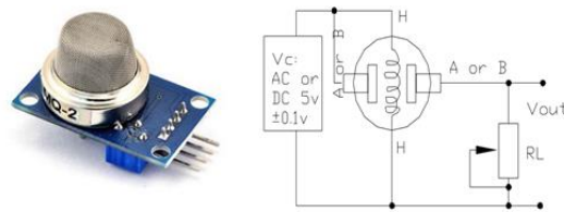
Fig 5. MQ-2 Sensor Module
